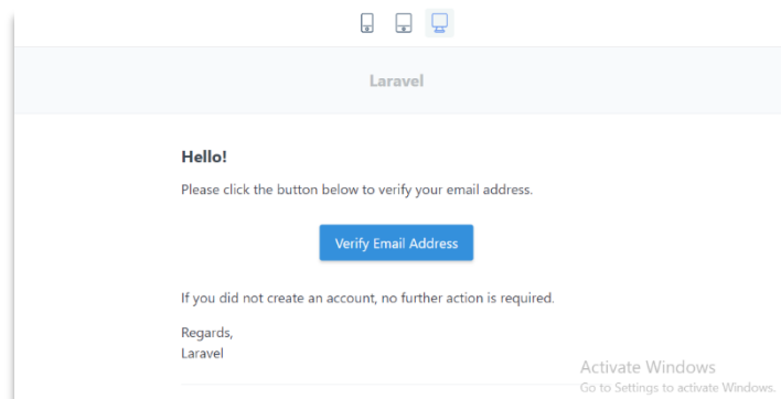
Gambar 6. Verifikasi Akun
